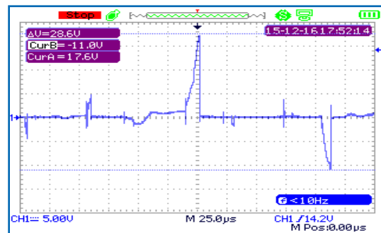
Messung der Wellenspannung eines Motors mit FU-Antrieb ohne einen AEGIS® Wellenerdungsring
