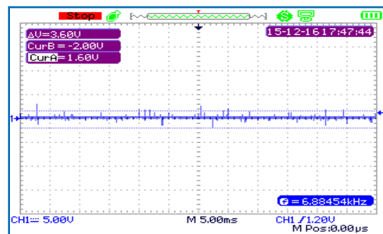
Messung der Wellenspannung eines Motors mit FU-Antrieb mit einem AEGIS® Wellenerdungsring
