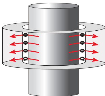
Elektronen-Tunneleffekt
