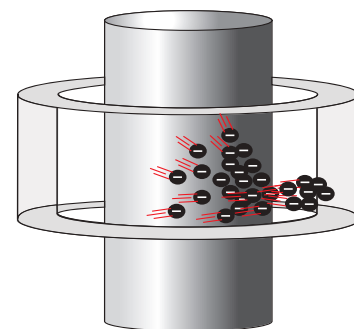
Townsend-Entladung von Gas-Ionen
